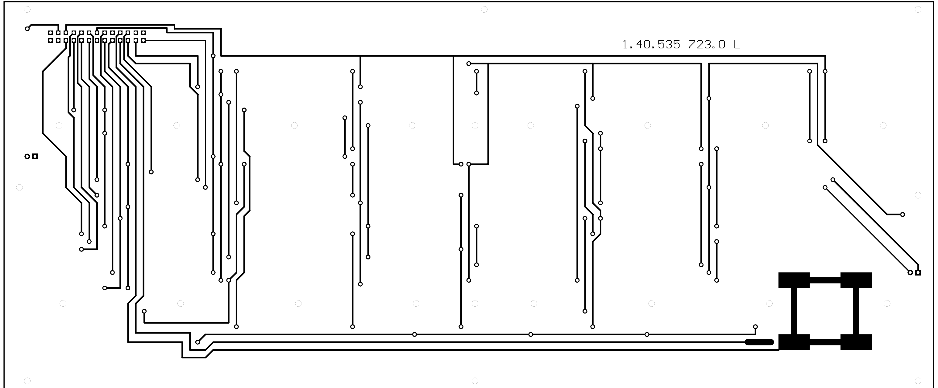
Leiterbild L-Seite
