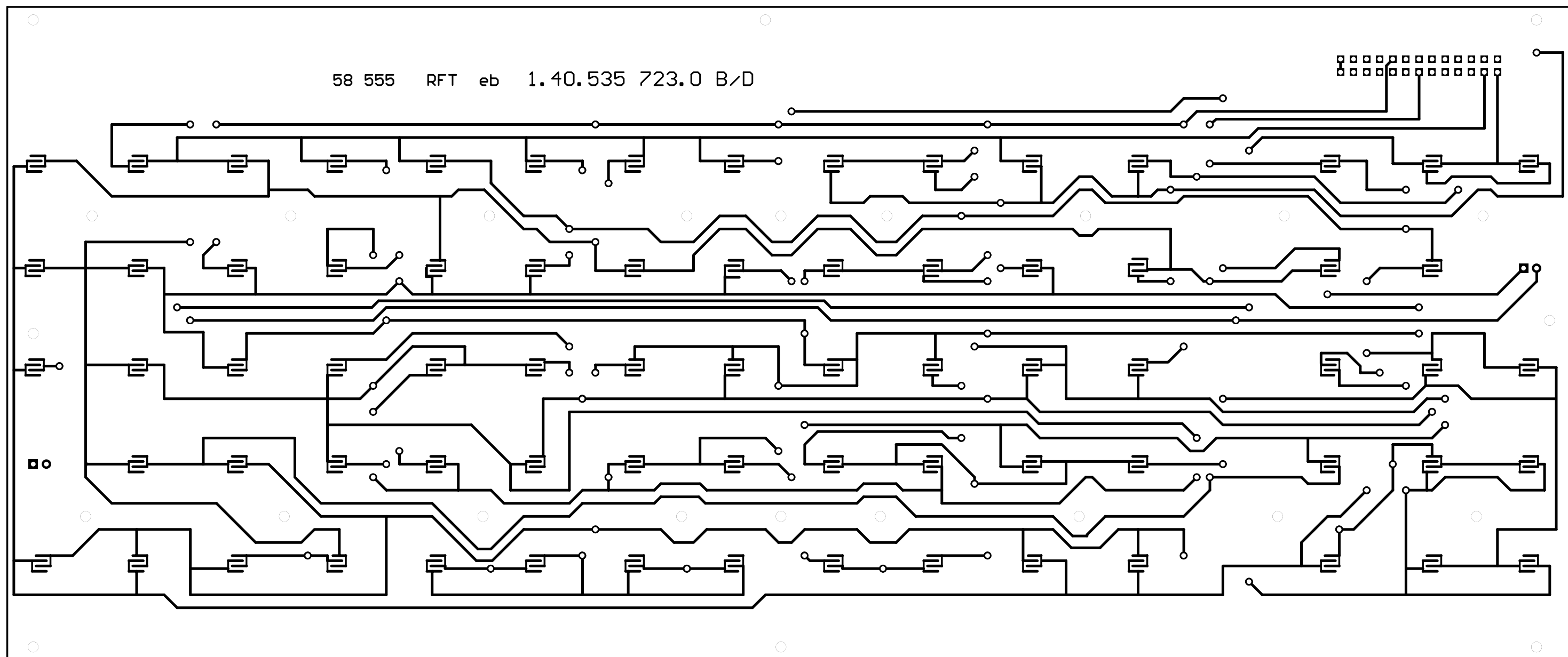
Leiterbild B-Seite
