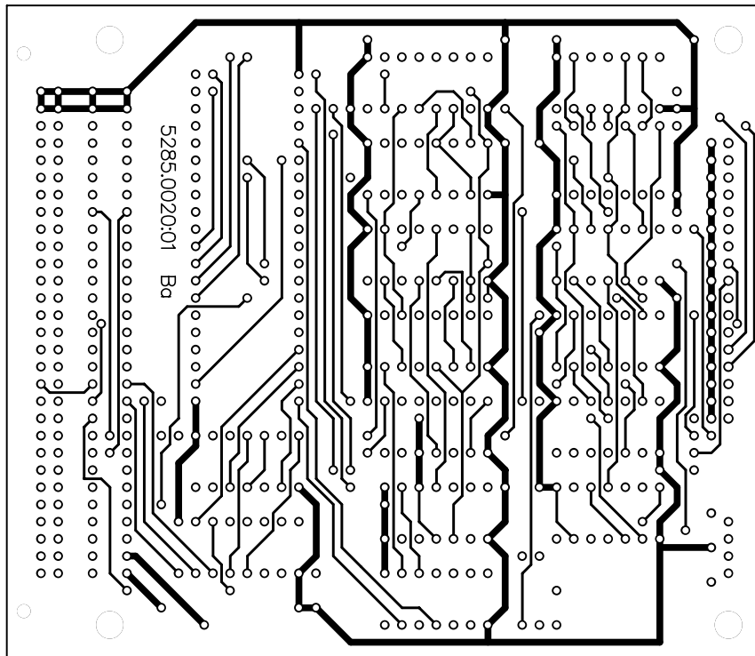
Top Layer
