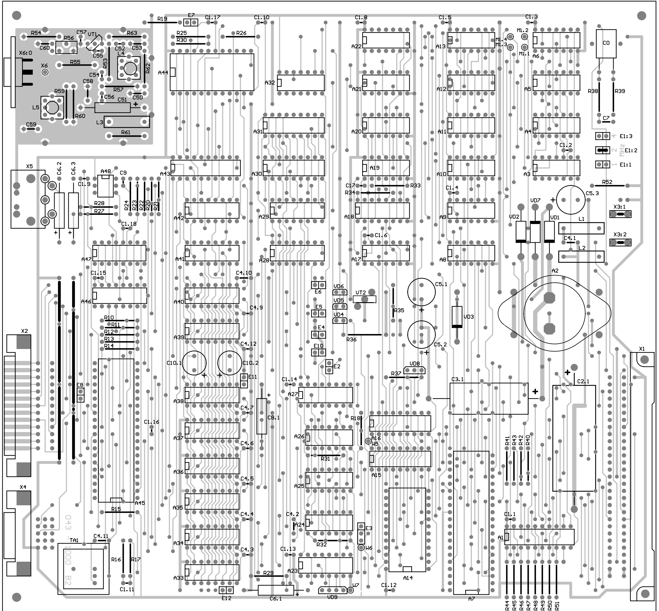
Lageplan Z1013.64
