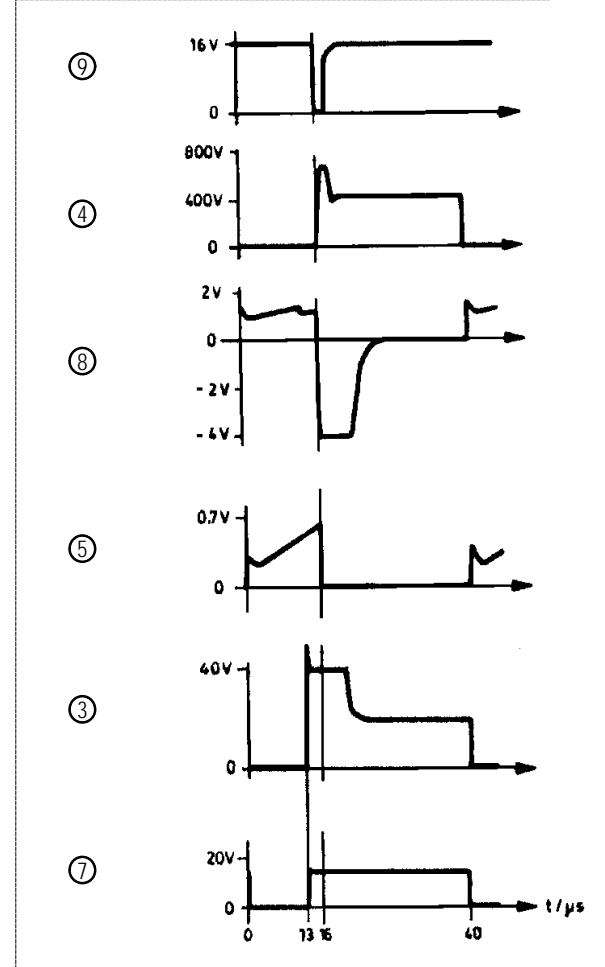
① Bezugswert für alle Spannungswerte und Oszillogramme Die Amplituden- und Zeitwerte der Oszillogramme beziehen sich auf 220V Netzspannung und 25W Ausgangsbelastung
