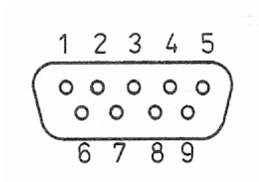
Bild 9: Steckerleiste JOYSTICK
