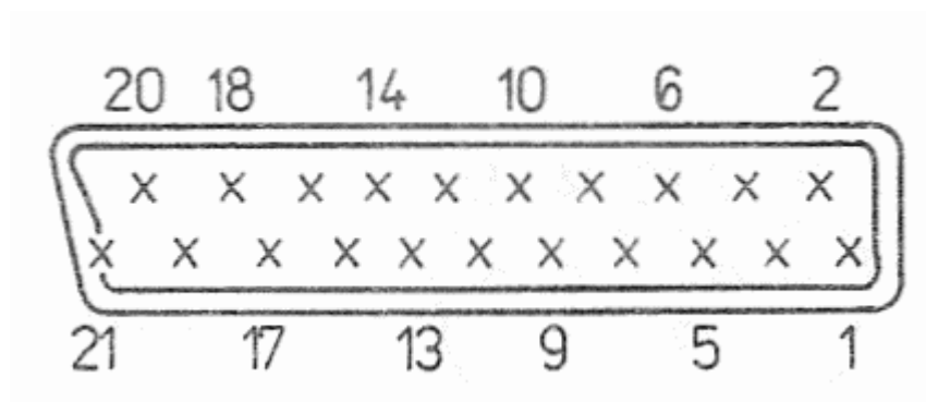
Bild 6: Buchsenleiste TV-RGB
