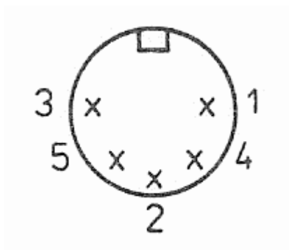
Bild 7: Diodenbuchse SOUND
